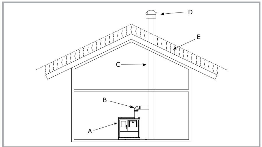
Abb. 3 - Teile des Kamins A = Holzherd, B = Rauchrohrstutzen, C = Rauchabzug, D = Schornstein, E = Windfangbereich.
