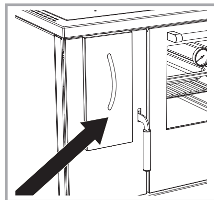
Figure 24 – Bouclier thermique sur la porte foyère.
