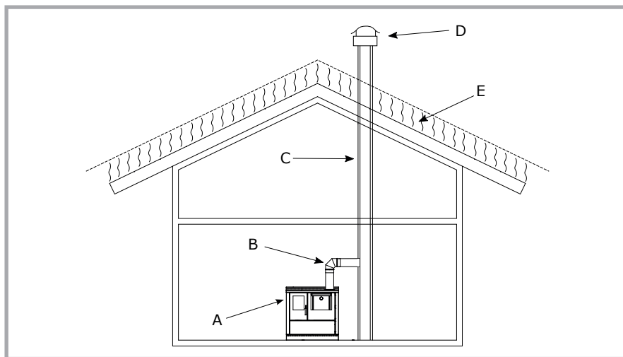
Figura 3 - Le parti componenti del camino. A= Cucina B= Raccordo o canale da fumo C= Canna fumaria D= Comignolo E= zona di riflusso
