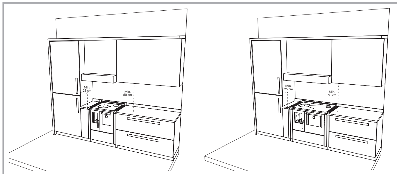
Abb. 2 - Mindestsicherheitsabstände für den Einbau, mit eigens dazu bestimmten Abstandsverbindungen zum Einbau neben hitzeempfindlichen Materialien.
