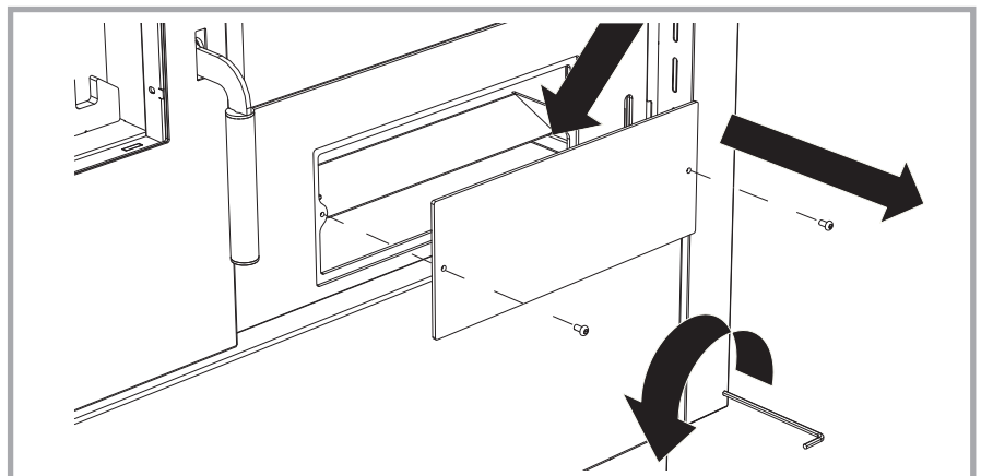
Abb. 26 - Reinigung der Rauchgaszüge
