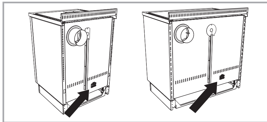
Figura 13 - Posizione della morsettiera per l'allacciamento alla rete elettrica.
