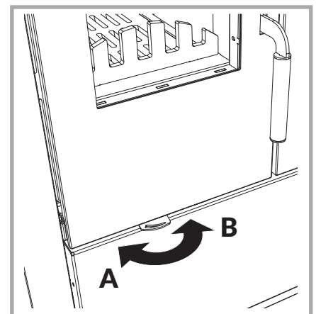
Abb. 19 - Einstellung der Luftzufuhr-Regulierung. Wenn sich der Hebel auf der Position "A" befindet, ist die Luftzufuhr offen. Auf der Position "B" ist die Luftzufuhr geschlossen.
