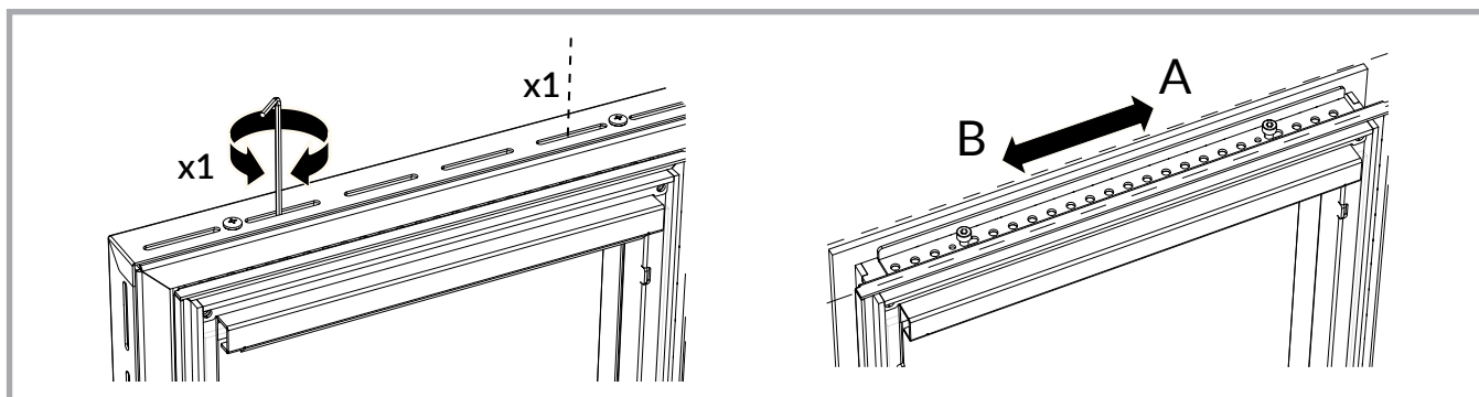
Figura 20 - Regolazione ausiliaria dell'aria per la pulizia del vetro: la piastrina è aperta in corrispondenza della posizione indicata con la lettera A, mentre è chiusa in corrispondenza della posizione indicata con la lettera B.
