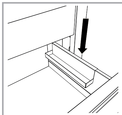
Abb. 22 - Im Inneren der Holzlade montiertes Zubehörfach.
