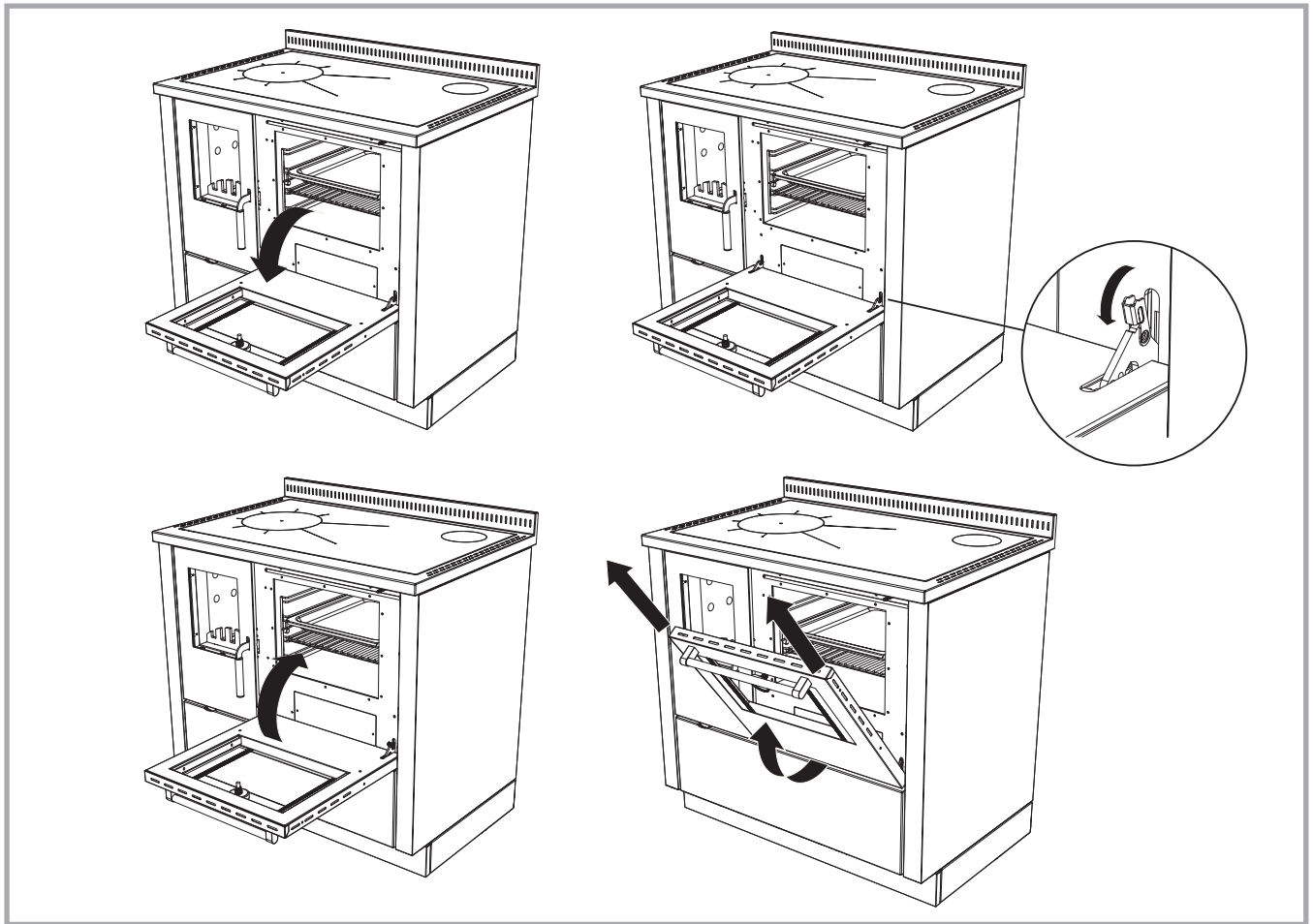
Abb. 25 - Entfernung der Backofentür
