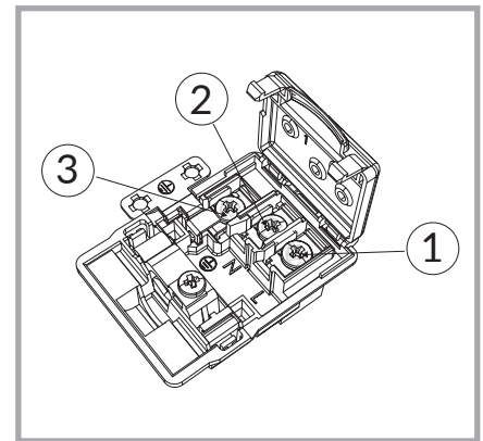
Abb. 14 - Klemmbrett für den Anschluss an die Stromversorgung: 1. Phase, 2. Neutralleiter, 3. Schutzleiter.
