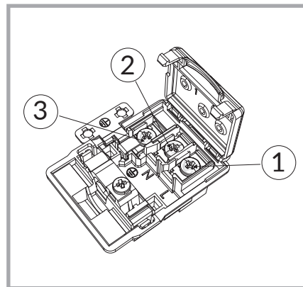
Figura 14 - Morsettiera elettrica per il collegamento alla rete: 1. Linea 2. Neutro 3. Terra
