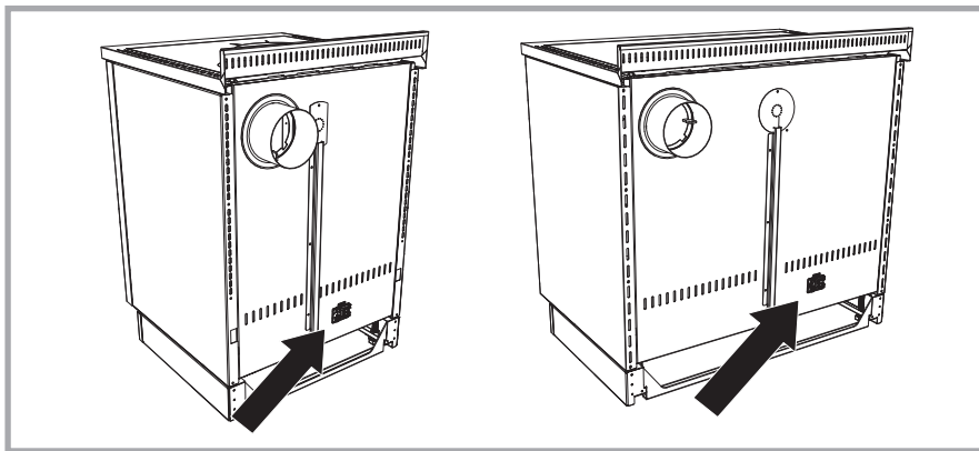
Abb. 13 - Position des Klemmbretts für den Anschluss an die Stromversorgung.
