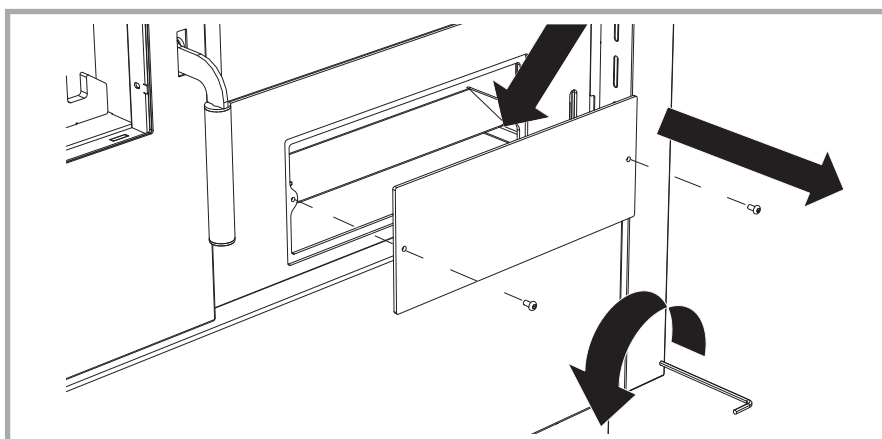
Figura 26 - Ispezione girofumi.
