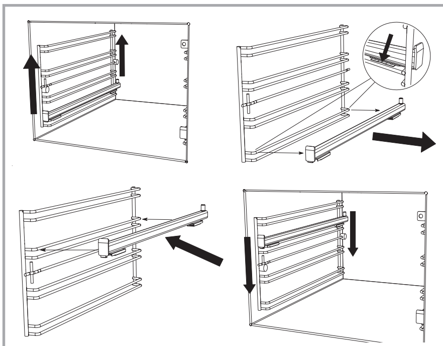
Abb. 29 - Vorgangsweise zum Umstecken des Teleskopauszugs.
