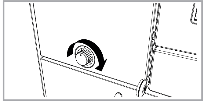
Figura 25 - Regolazione dell'aria primaria e secondaria. Il regolatore si apre ruotando la manopola in senso orario.
