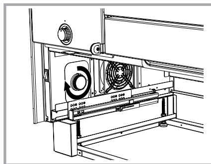
Abb. 28 - Thermostateinstellung für die Zwangslüftung der Seitenwände.
