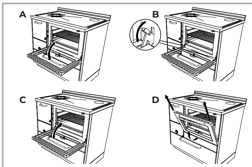
Abb. 34 - Aushängen der Backofentür.
