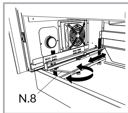
Figura 21 - Regolazione della rientranza dello zoccolo rispetto al corpo della cucina.
