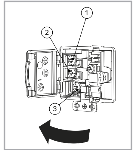
Figura 19 - Morsettiera elettrica per il collegamento alla rete: 1. Linea 2. Neutro 3. Terra
