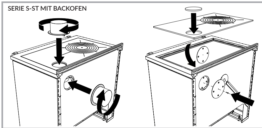
Abb. 8 – Mehrfachanschluss für Holz- und Zentralheizungsherde mit Backofen, korrekte Vorbereitung für den Anschluss.
