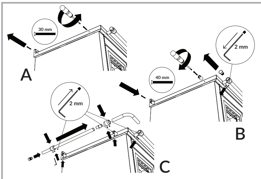
Abb. 20 - Montage der Herdstange.
