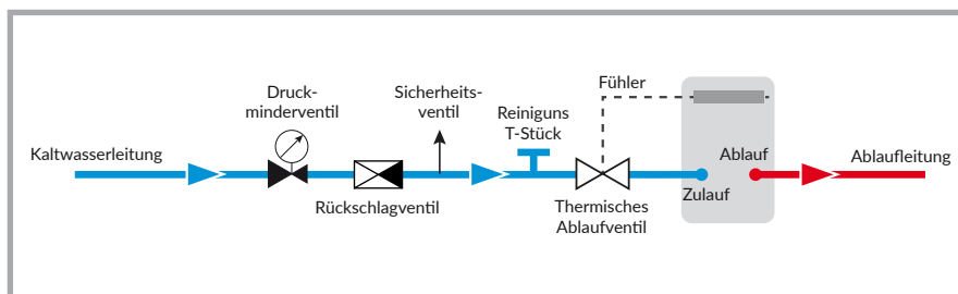
Abb. 23 – Schematische Darstellung für den Kreislauf des Sicherheitswärmetauschers.
