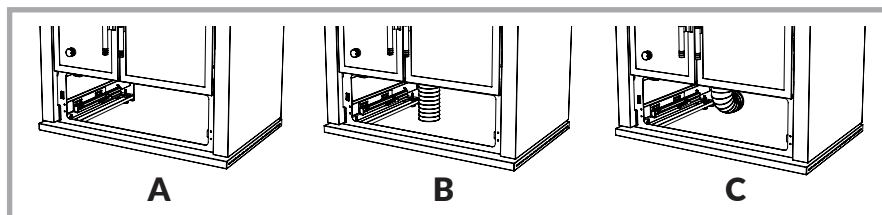
Abb. 14 – Anschlussmöglichkeiten der Frischluftzufuhr am Holzherd. A = Externe Frischluftzufuhr nicht angeschlossen, B = Externe Frischluftzufuhr Anschluss in Bodenhöhe, C = Externe Frischluftzufuhr Wandanschluss.
