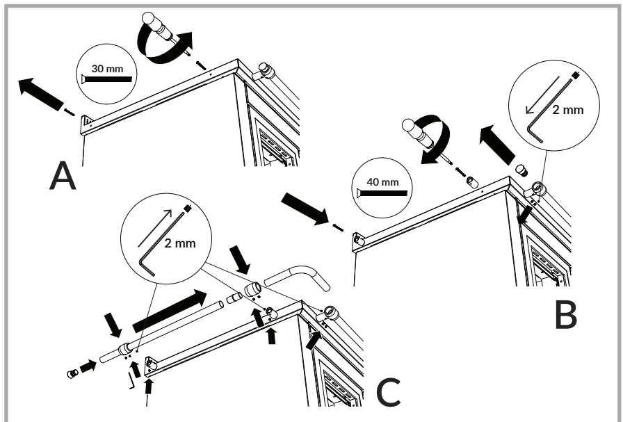
Figura 20 - Modifica del corrimano.
