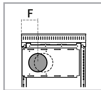
Abb. 12a – Rückansicht des Gerätes und Darstellung der min. und max. Verschiebung des Rauchausgangs auf der Rückseite mit der Standard-Anschlussplatte.
