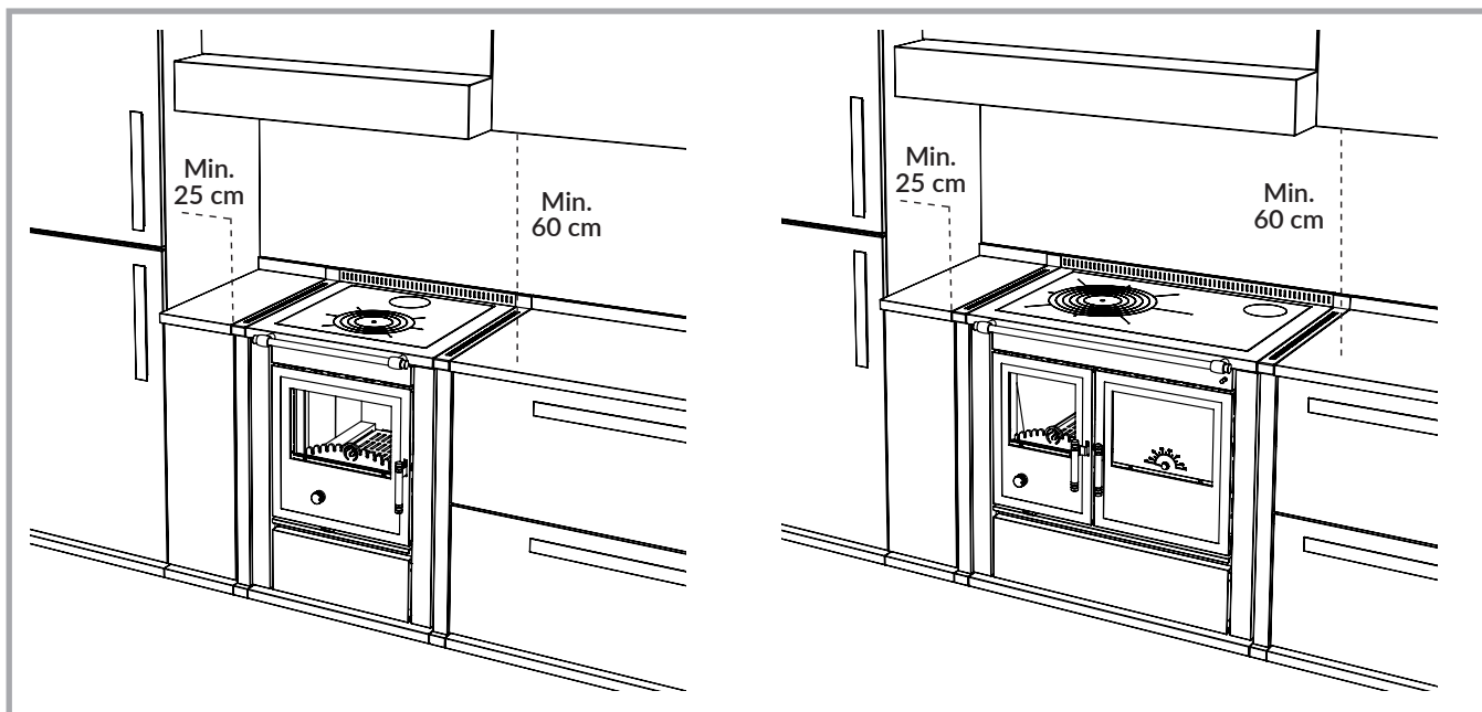
Figura 3 - Distanze minime di sicurezza in abbinamento ad appositi distanziatori per l'inserimento ad incasso.
