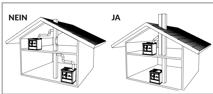
Abb. 5 – Beispiel für falsche und richtige Ausführung des Rauchabzugs.
