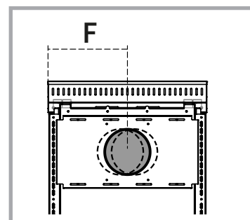
Figura 12b - Vista posteriore dell'apparecchio e rappresentazione dello spostamento minimo e massimo riguardo la posizione dell'uscita fumi posteriore con la lamiera aggiuntiva.
