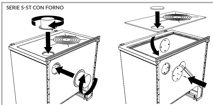
Figura 8 - Cucina o termocucina multifuelo con forno, predisposizione dell'uscita fumi corretta.
