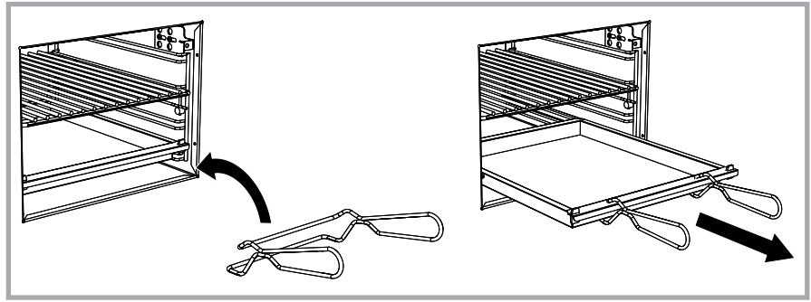
Abb. 36 – Backblechhalter.
