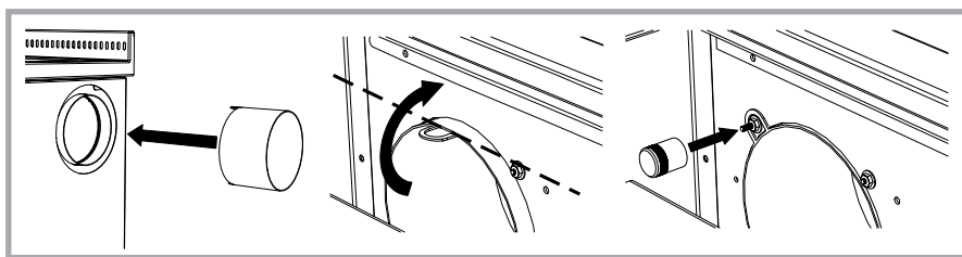
Figura 11 - Uscita fumi sul fianco. Fissaggio del connettore per uscita fumi sul fianco.
