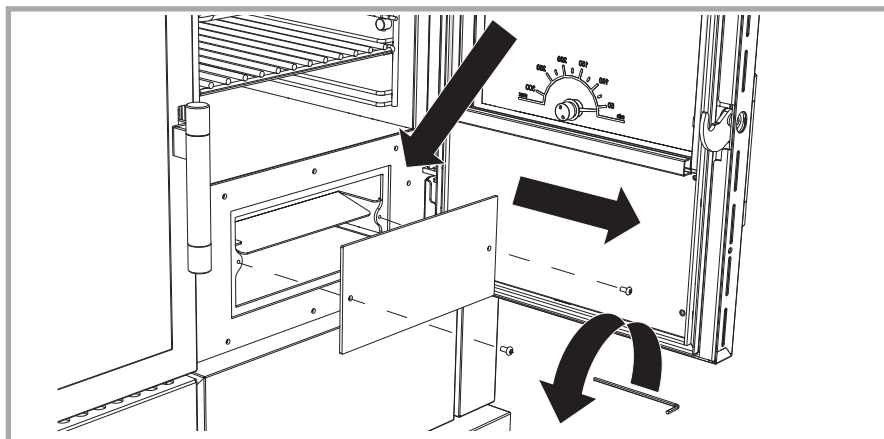
Abb. 48 – Kontrolle der Rauchgaszüge.
