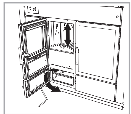
Abb. 41 - Höhenverstellbarer Feuerrost.
