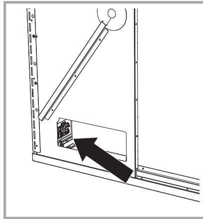
Abb. 14 – Position des Klemmbretts für den Anschluss an die Stromversorgung.
