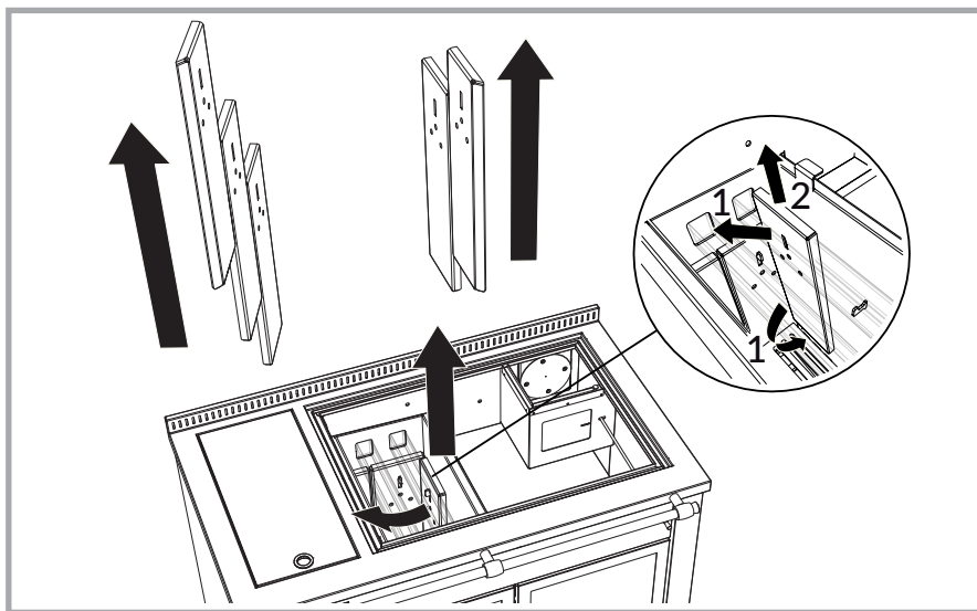
Abb. 47 – Wartung der Metallplatten in der Brennkammer.
