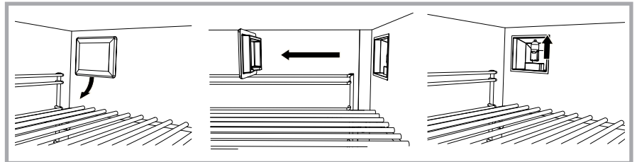
Abb. 49 – Austausch der Backofenlampe
