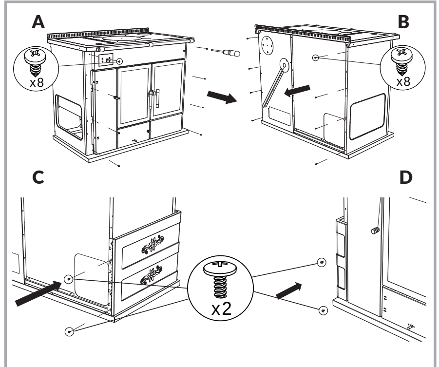
Abb. 13 – Position der Schrauben am Zentralheizungsherd um die Seitenwände korrekt anzubringen und Befestigung der Elemente der Seitenwände.
