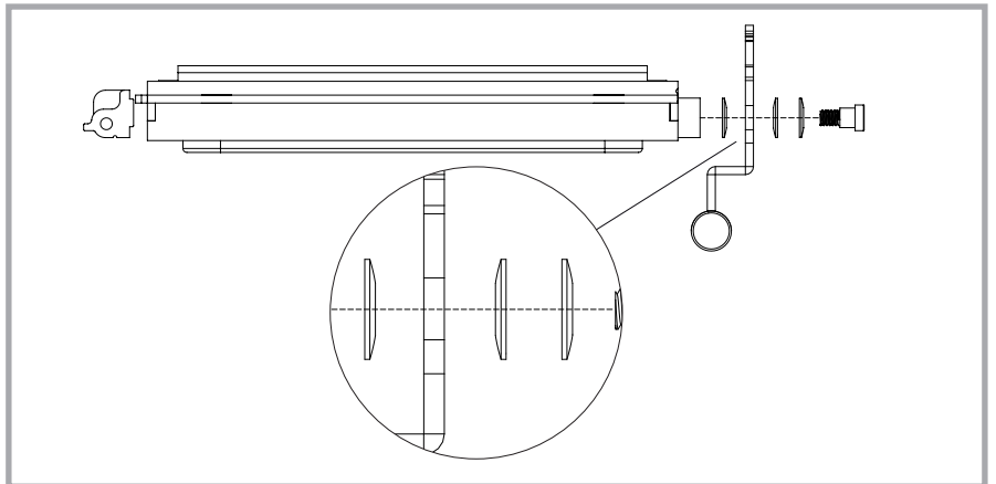
Abb. 50 – Korrekte Position der Kegelscheiben
