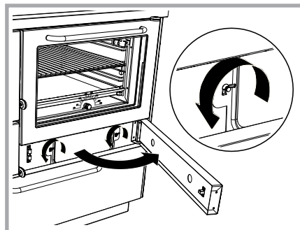
Figura 32 - Ispezione girofumi.
