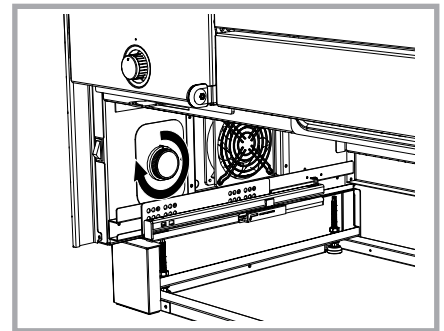
Abb. 28 - Thermostateinstellung für die Zwangselüftung der Seitenwände.
