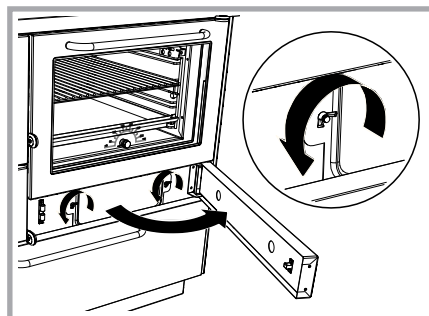
Abb. 32 - Kontrolle der Rauchgaszüge.
