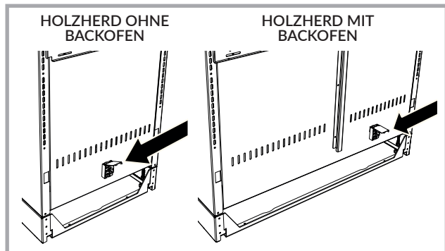
Abb. 17 - Position des Klemmbretts für den Anschluss an die Stromversorgung.
