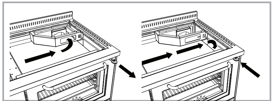
Abb. 23 - Anheizklappen-Hebel. Bei herausgezogenem Hebel ist die Klappe offen und das Anheizen ist einfacher. Bei nicht herausgezogenem Hebel ist die Klappe für den Normalbetrieb geschlossen.
