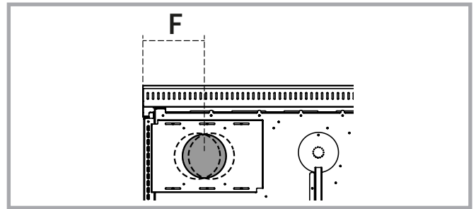
Abb. 13c - Rückansicht des Holzherdes und Darstellung der min. und max. Verschiebung des Rauchausgangs auf der Rückseite mit der zusätzlichen Anschlussplatte.
