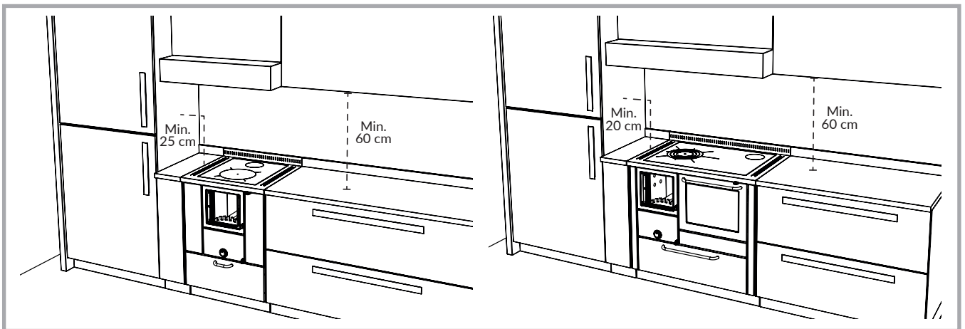
Figura 3 – Distanze minime di sicurezza per l'inserimento ad incasso delle cucine serie RI - RVI in prossimità di materiale infiammabile.
