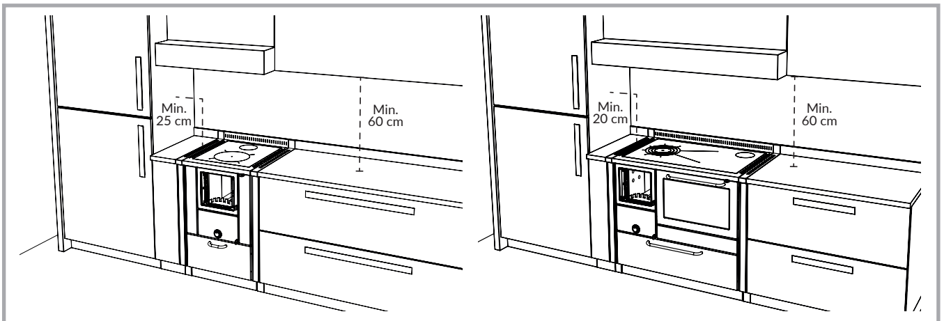
Figura 2 – Distanze minime di sicurezza in abbinamento ad appositi distanziatori per l'inserimento ad incasso delle cucine serie RE - RVE in prossimità di materiale infiammabile.
