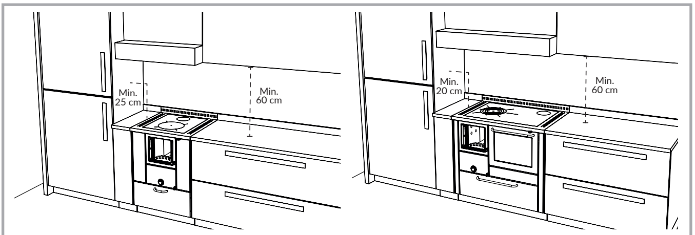
Abb. 3 - Mindestsicherheitsabstände für den Einbau der Holzherde Serie RI - RVI neben hitzeempfindlichen Materialien.
