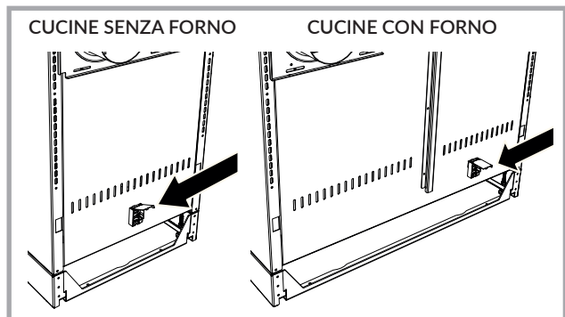
Figura 17 - Posizione della morsettiera per l'allacciamento alla rete elettrica.
