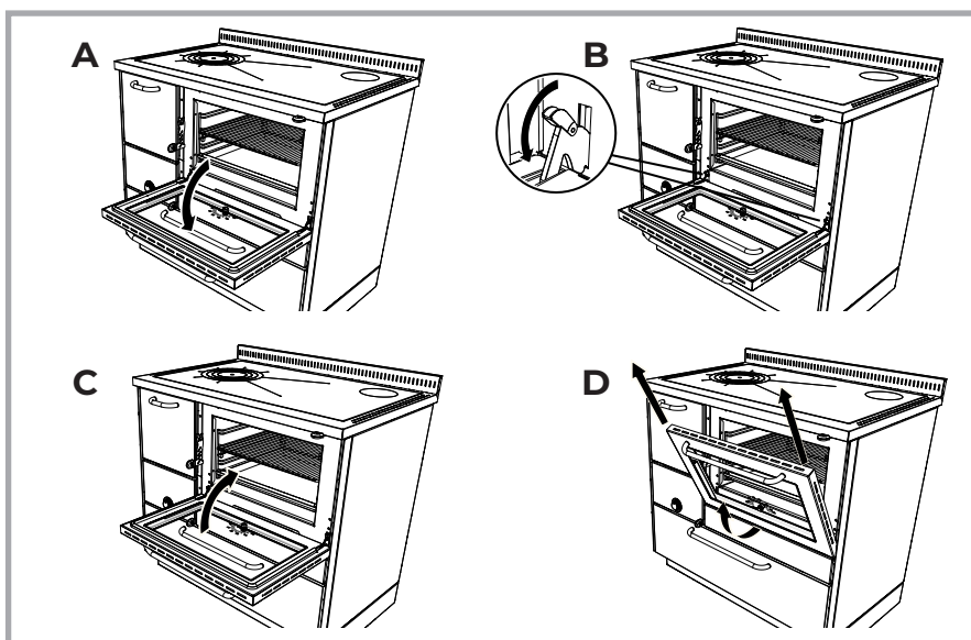
Abb. 33 - Aushängen der Backofentür.
