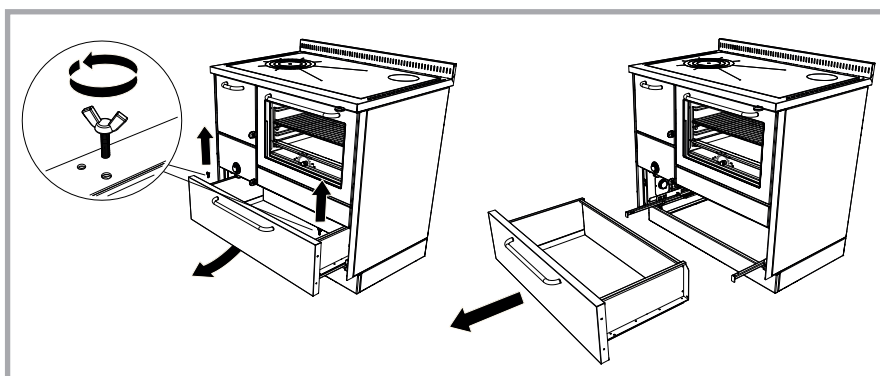
Abb. 19 - Entfernung der Holzlade.
