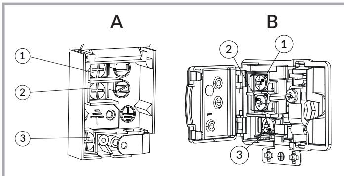
Abb. 18 - Klemmbrett für den Anschluss an die Stromversorgung: 1. Phase, 2. Neutralleiter, 3. Schutzleiter.
