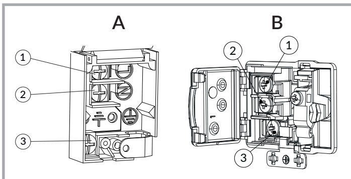
Figura 18 - Morsettiera elettrica per il collegamento alla rete: 1. Linea 2. Neutro 3. Terra
