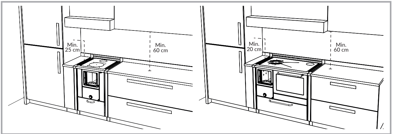
Abb. 2 - Mindestsicherheitsabstände für den Einbau, mit eigens dazu bestimmten Abstandsverbindungen zum Einbau der Holzherde Serie RE - RVE neben hitzeempfindlichen Materialien.
