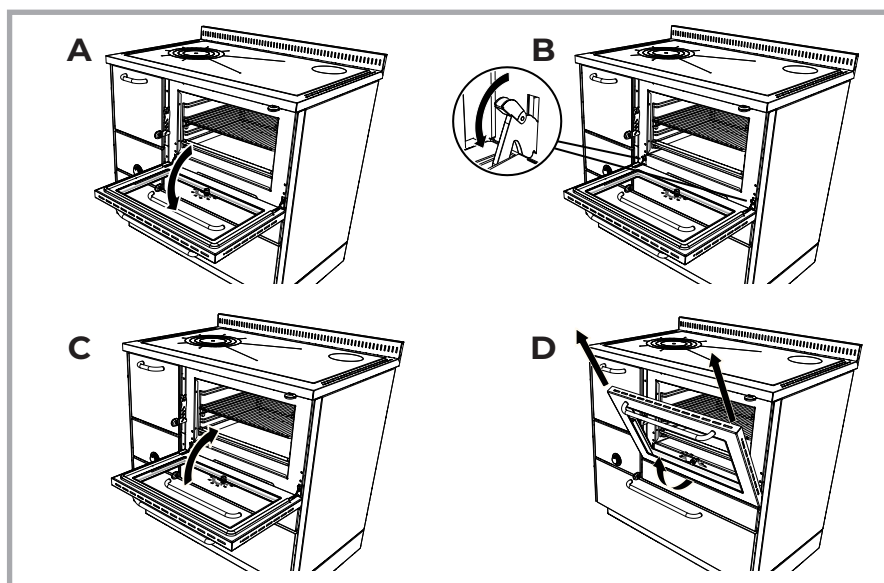
Figura 33 - Smontaggio della porta forno.
