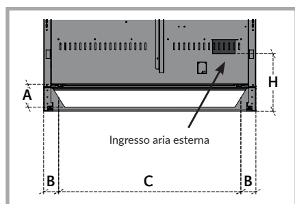
Figura 16 - Vista posteriore dello zoccolo della cucina a legna e specifiche per il collegamento con la presa d'aria esterna.
