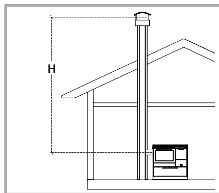
Abb. 6 - Maß H für Bemessung des Rauchabzugsrohrs.
