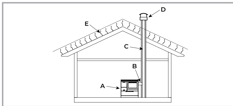
Figura 4 - Le parti componenti del camino. A= Cucina B= Raccordo o canale da fumo C= Canna fumaria D= Comignolo E= zona di riflusso
