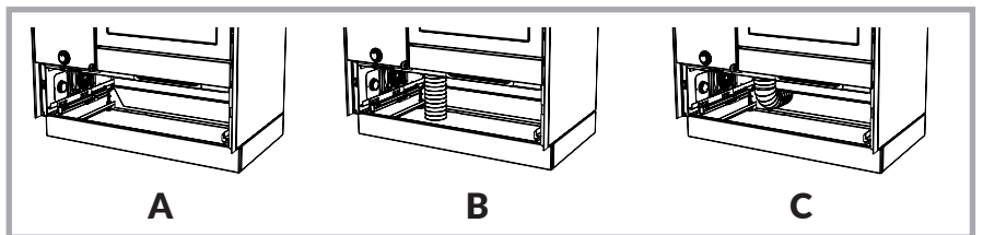
Abb. 15 - Anschlussmöglichkeiten der Frischluftzufuhr am Holzherd. A = Externe Frischluftzufuhr nicht angeschlossen, B = Externe Frischluftzufuhr Anschluss in Bodenhöhe, C = Externe Frischluftzufuhr Wandanschluss
