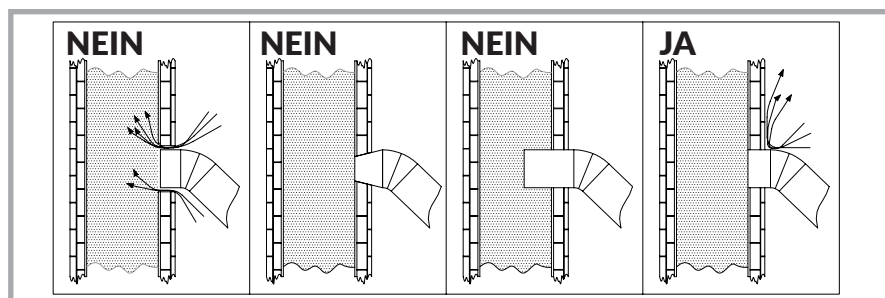
Abb. 11 - Beispiele für den richtigen und falschen Anschluss an das Rauchabzugsrohr.
