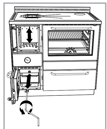
Abb. 32 - Höhenverstellbarer Feuerrost
