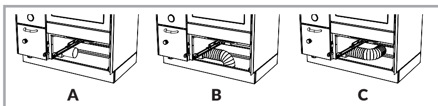
Figura 13 - Modi di collegamento della presa d'aria della termocucina a legna. A= Presa aria esterna non collegata, B= Presa aria esterna al pavimento, C= Presa aria esterna a parete.
