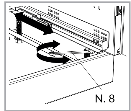
Abb. 19 - Einstellung des Sockeleinzugs.
