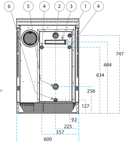
Abb. 20 - Anschlusschema der Modelle RTE 60 und RTVE 60 mit Rauchausgang rechts (Rückansicht). Bei Modellen mit Rauchausgang links befinden sich die Anschlüsse symmetrisch.
