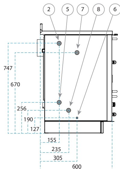
Abb. 22 - Anschlusschema der Modelle RTE / RTVE mit seitlichen Anschlüssen (Seitenansicht).
