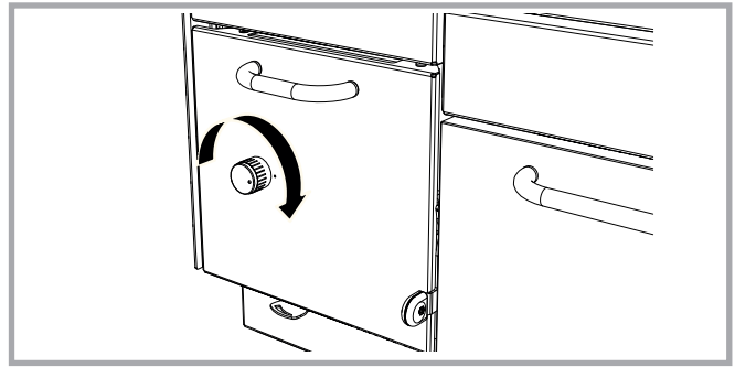
Abb. 30 - Einstellung der Primärluft. Durch das Drehen im Uhrzeigersinn, öffnet sich die Regulierung.
