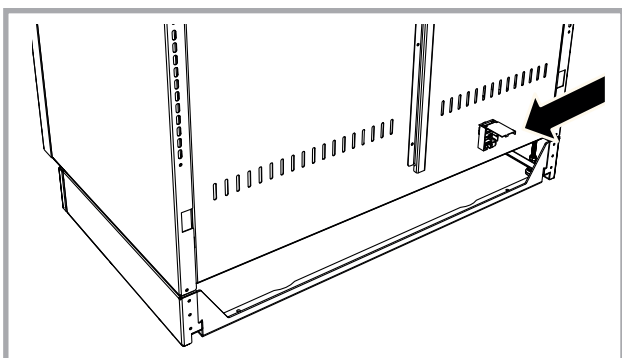
Figura 15 - Posizione della morsettiera per l'allacciamento alla rete elettrica.
