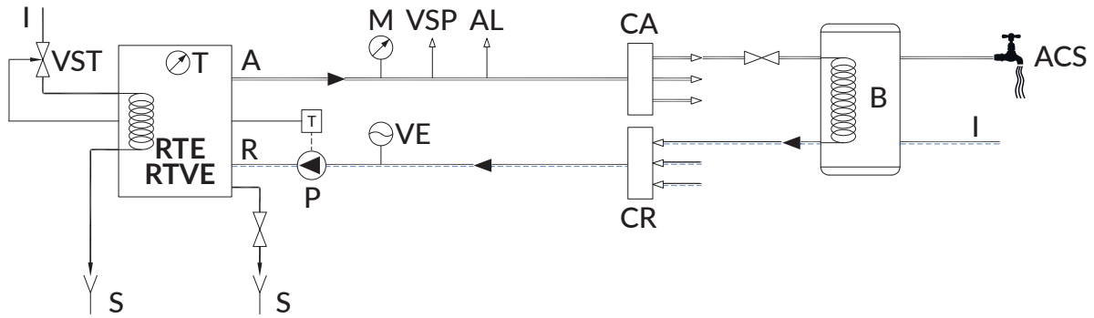
Abb. 26 - Beispiel einer Heizungsanlage mit Zentralheizungsherd als Wärmeerzeuger.
