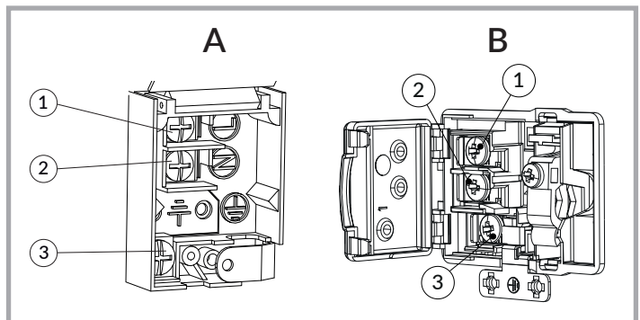
Abb. 16 - Klemmbrett für den Anschluss an die Stromversorgung: 1. Phase, 2. Neutraleiter, 3. Schutzleiter.
