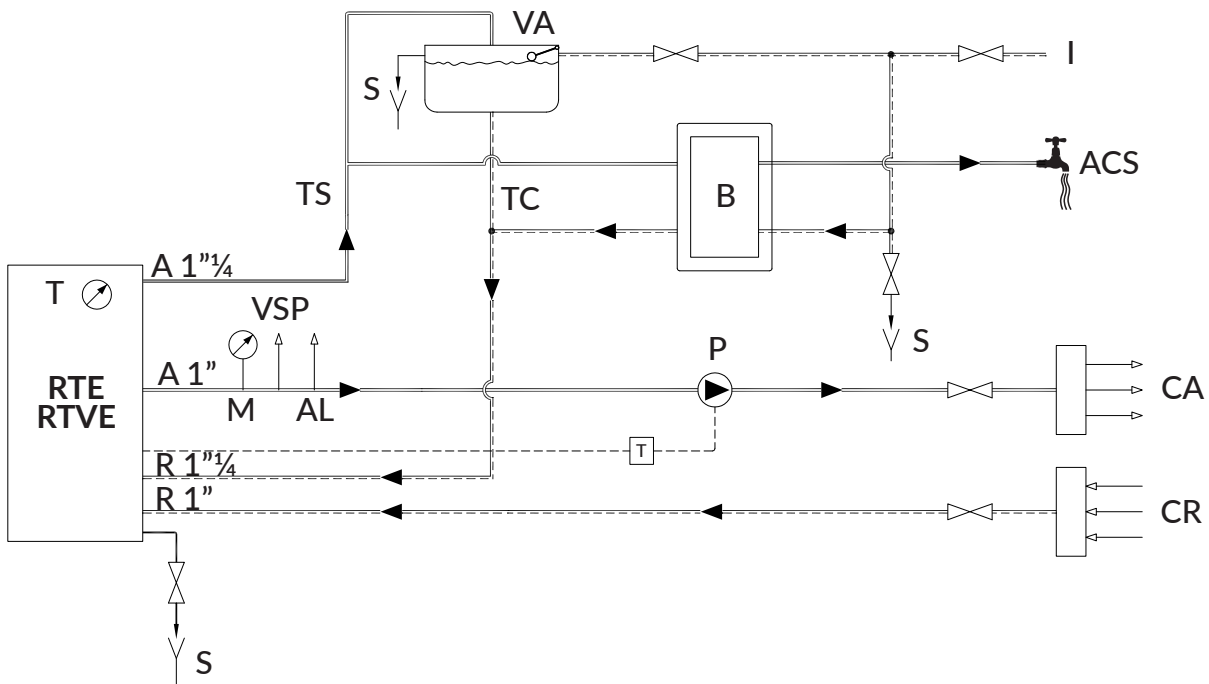
Abb. 27 - Beispiel einer Heizungsanlage mit Zentralheizungsherd mit doppelten Anschlüssen (Serie RTE-RTVE mit seitlichen Anschlüssen) als Wärmeerzeuger.
