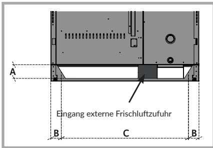
Abb. 14 - Rückansicht des Sockels und Angaben für den Anschluss an die externe Frischluftzufuhr.
