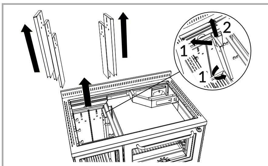
Figura 38 – Manutenzione delle lamiere in camera di combustione
