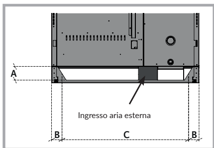
Figura 14 - Vista posteriore dello zoccolo della termocucina e specifiche per il collegamento con la presa d'aria esterna.
