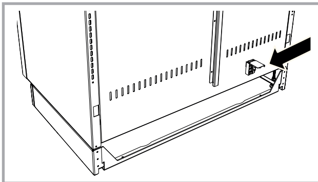
Abb. 15 - Position des Klemmbretts für den Anschluss an die Stromversorgung.
