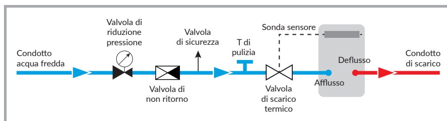
Figura 23 - Schema realizzativo del circuito di scarico termico.
