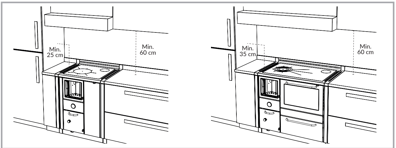
Abb. 2 - Mindestsicherheitsabstände für den Einbau mit eigens dazu bestimmten Abstandsverbindungen.
