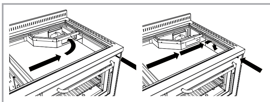
Abb. 28 - Anheizklappen-Hebel. Bei herausgezogenem Hebel ist die Klappe offen und das Anheizen ist einfacher. Bei nicht herausgezogenem Hebel ist die Klappe für den Normalbetrieb geschlossen.
