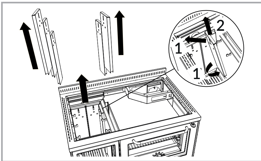
Abb. 38 - Wartung der Metallplatten in der Brennkammer.
