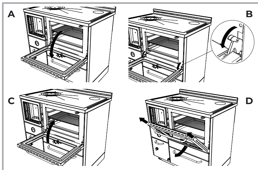
Figura 40 – Smontaggio della porta forno.
