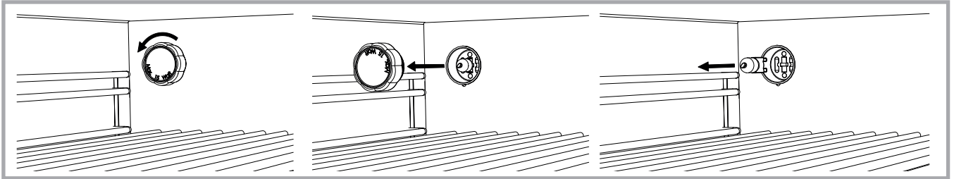
Abb. 41 - Austausch der Backofenlampe.
