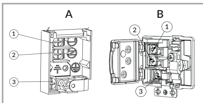
Figura 16 - Morsettiera elettrica per il collegamento alla rete: 1. Linea 2. Neutro 3. Terra
