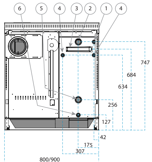
Abb. 21 - Anschlusschema der Modelle RTE 80, RTVE 80, RTE 90 und RTVE 90 mit Rauchausgang rechts (Rückansicht). Bei Modellen mit Rauchausgang links befinden sich die Anschlüsse symmetrisch.
