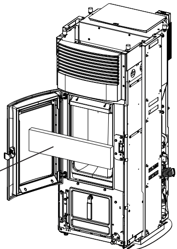
ENTFERNEN DES POLYSTYROL AUS DEM FEUERRAUM
