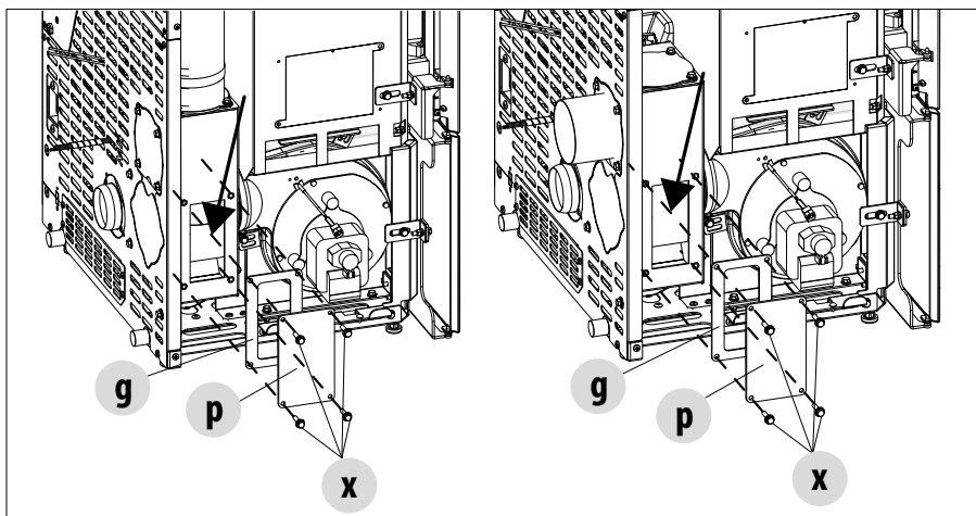
REINIGUNG DES OBEREN RAUCHAUSLASSES
