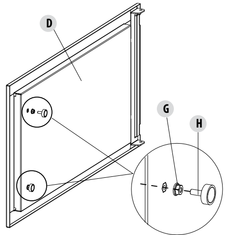
VERKLEIDUNG „METAL NERO“
