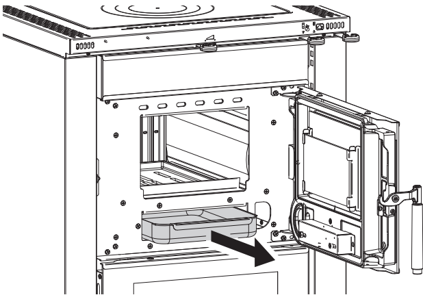
1 - ASCHESCHUBLADE
