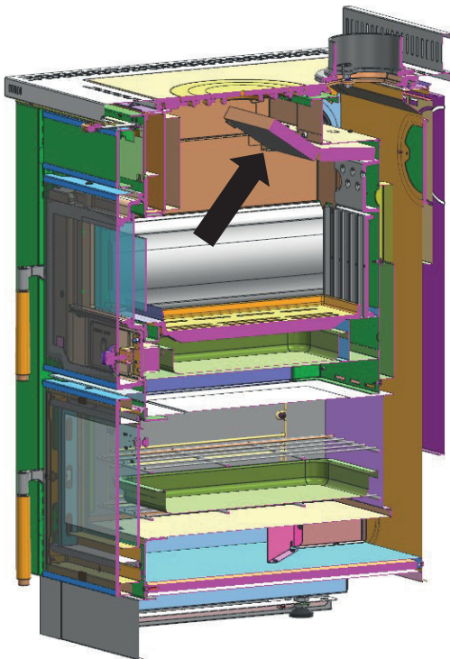
2 - RAUCHGASABWEISER
