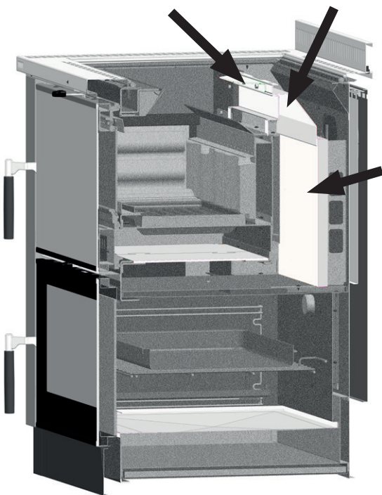
2 - RAUCHGASABWEISER
