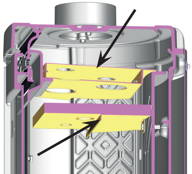
2 - RAUCHGASABWEISER
