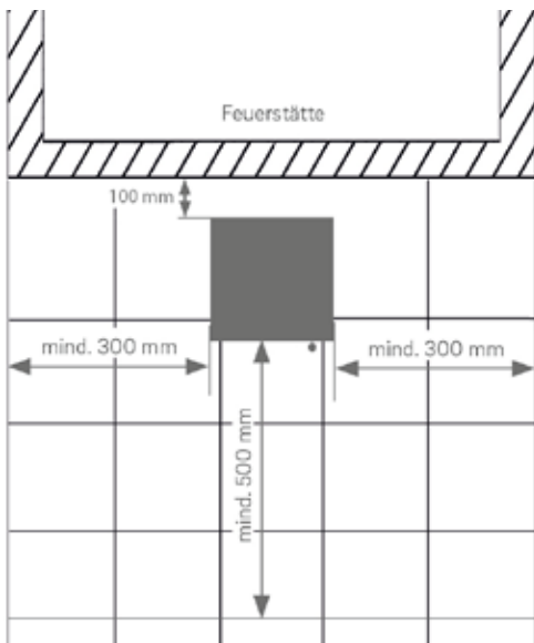
Abb.: 2 Fußbodenschutz im Bereich vor der Feuerraumöffnung
