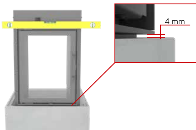
11. Grundofenkorpus mit Wasserwaage ausrichten und über die Revisionsöffnung ggf. nachstellen.
