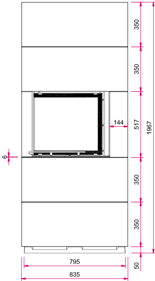
Frontansicht
