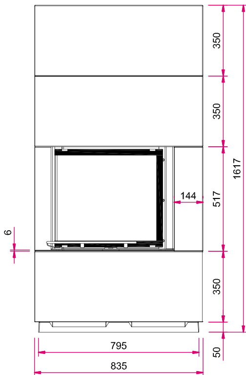
Frontansicht
