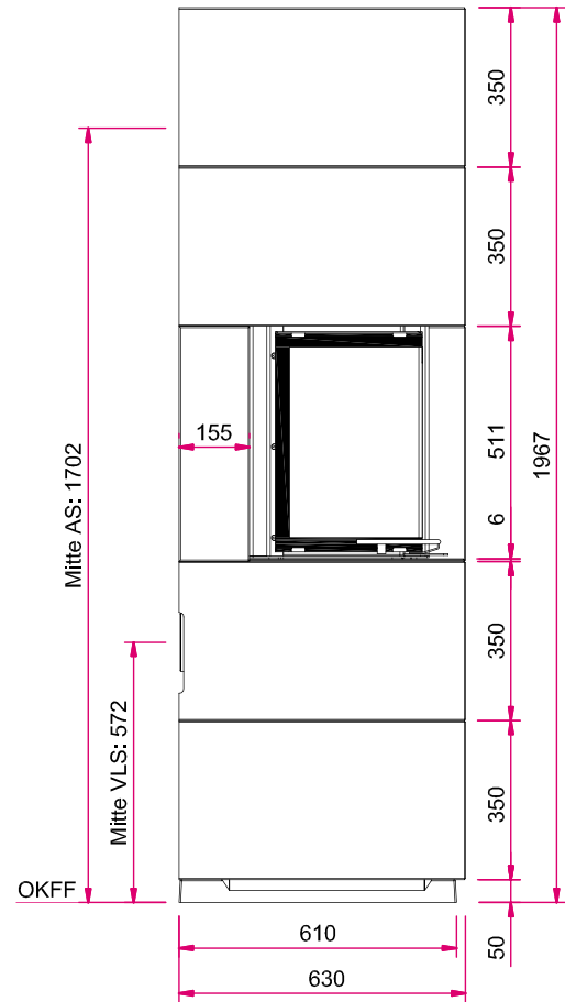
Seitenansicht
