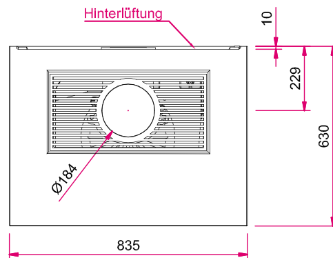
Draufsicht
