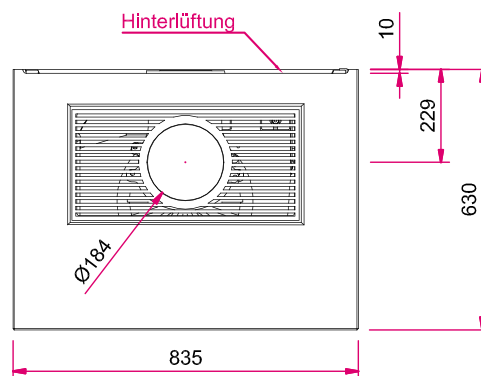
Draufsicht
