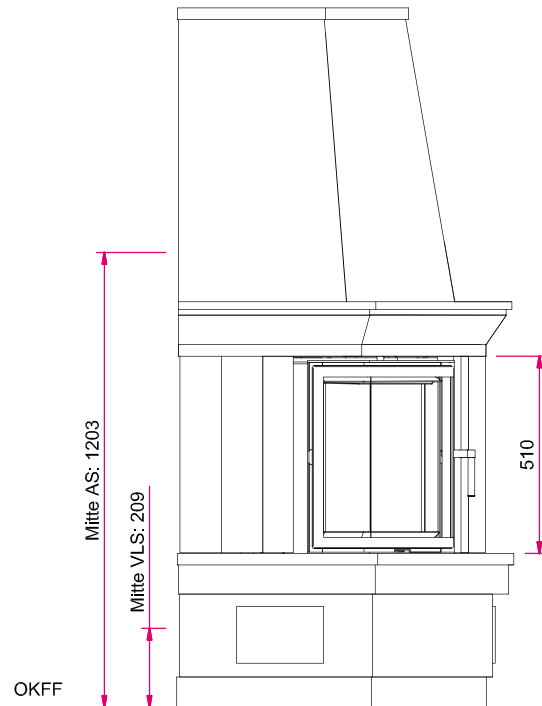
Seitenansicht links M 1:20
