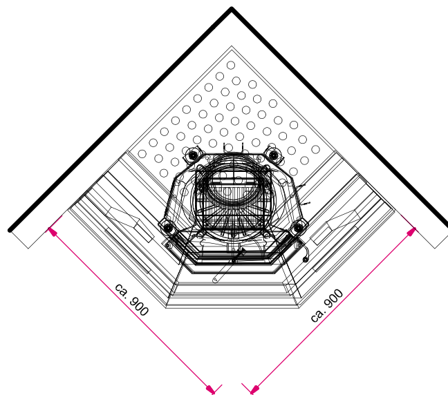
Draufsicht M 1:20
