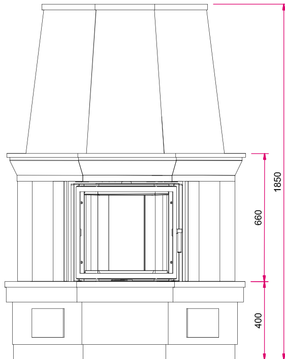
Frontansicht M 1:20
