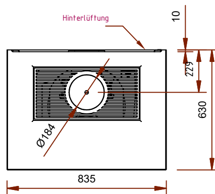
Draufsicht M 1:20
