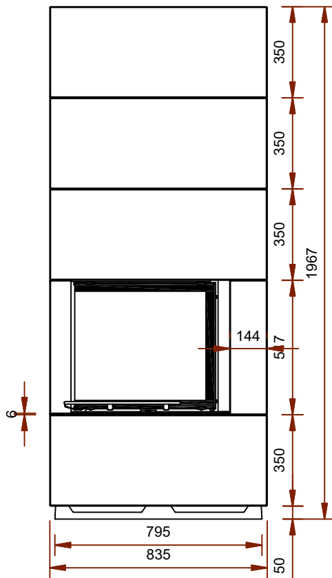
Frontansicht M 1:20
