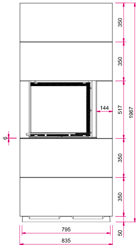
Frontansicht M 1:20
