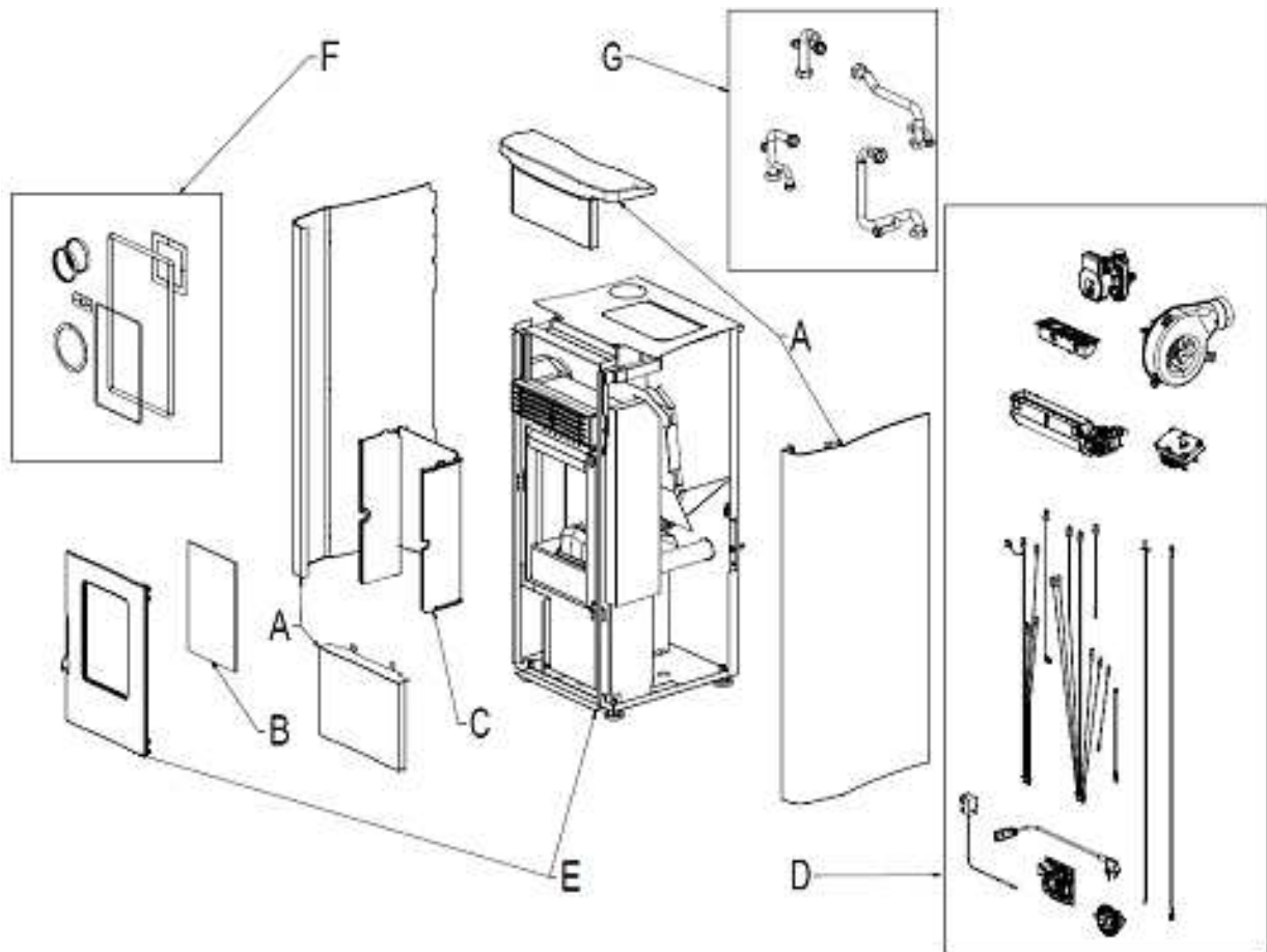
Fig. 1 - Explosionszeichnung
