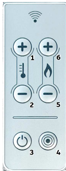
Fig. 33 - Fernsteuerung
