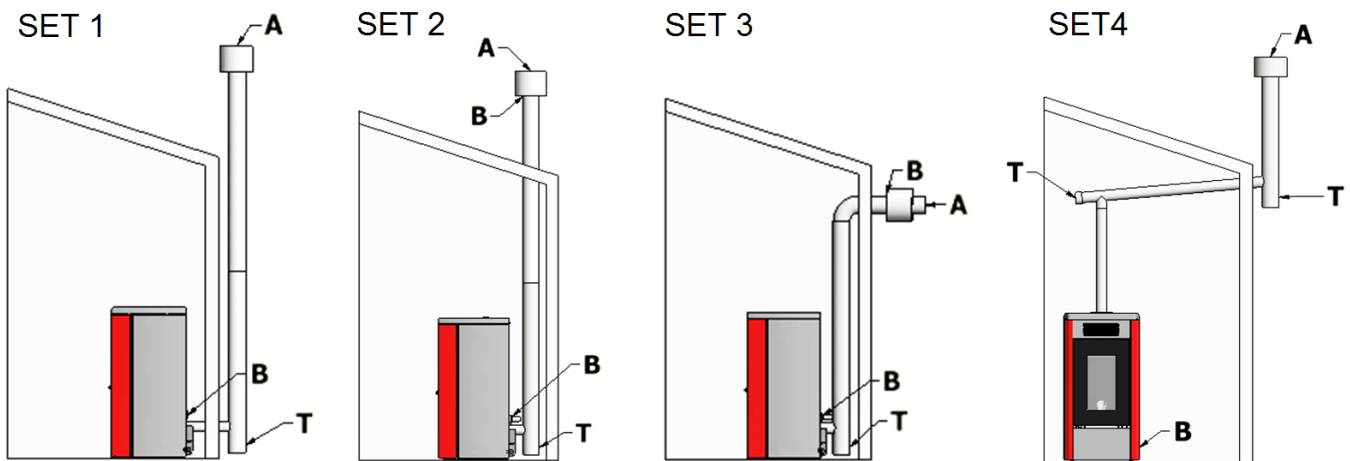
Fig. 23 - Beispiele festgelegt
