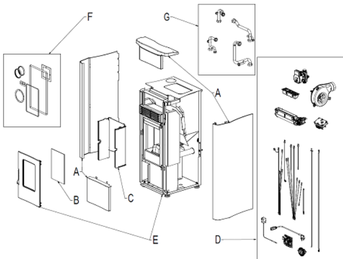
Fig. 1 - Explosionszeichnung
