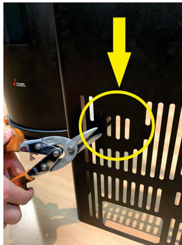
Fig. 61 - Ring zerschneiden
