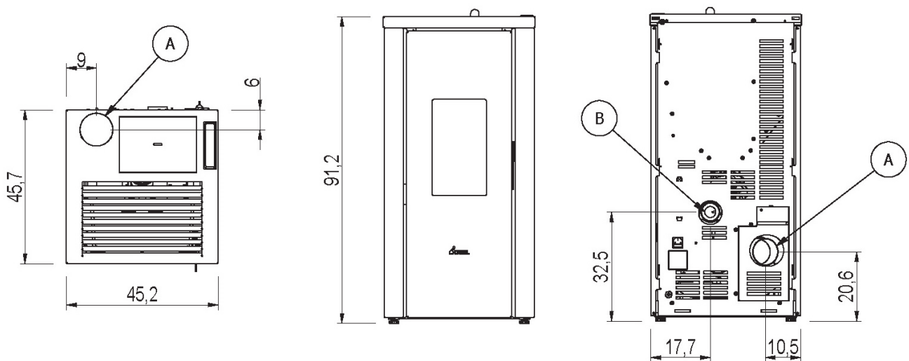
Fig. 25 - Allgemeine Abmessungen: VERA 7UP
