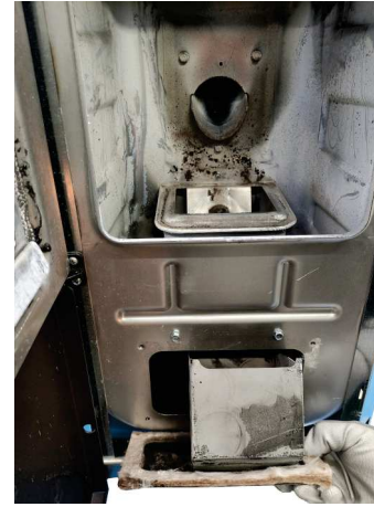
Fig. 78 - Den Inspektionsstopfen entfernen
