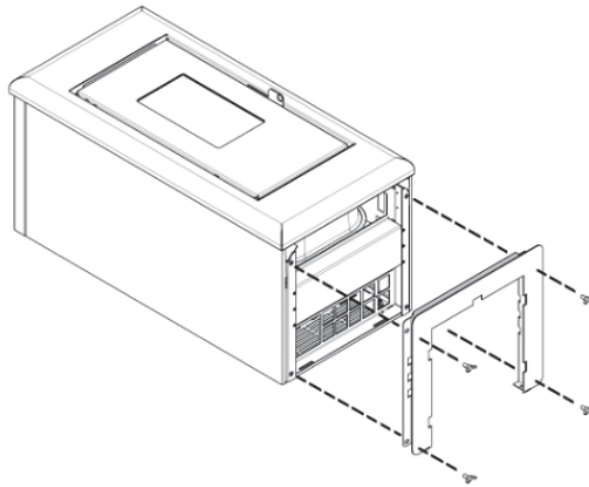
Fig. 50 - Montage des Sockels
