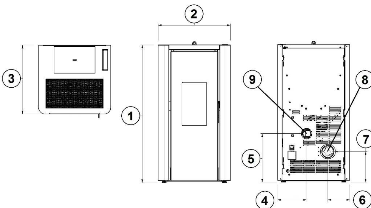
Fig. 24 - Allgemeine Abmessungen: INDIG07
