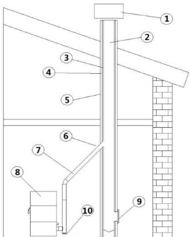
Fig. 2 - Bauteile Kamin
