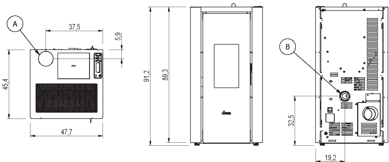
Fig. 26 - Allgemeine Abmessungen: CRISTAL 7UP
