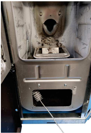
Fig. 79 - Mit einer Rohrreinigungsbürste reinigen
