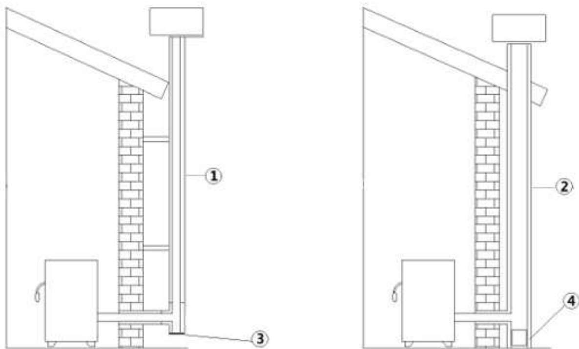
Fig. 3 - Rauchabzüge
