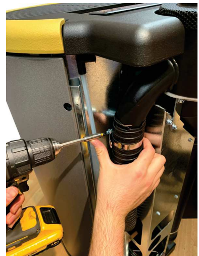
Fig. 62 - Schlauch herausziehen
