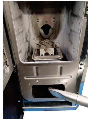
Fig. 80 - Die Asche absaugen
