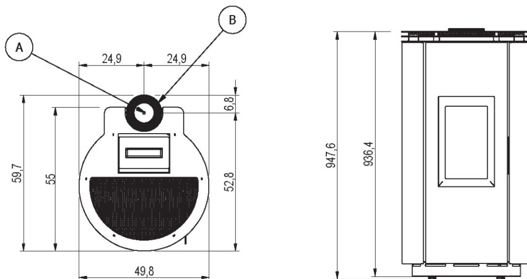
Fig. 19 - Allgemeine Abmessungen: FLOYD 5 - 7 - LORD 7
