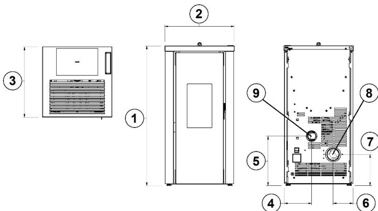
Fig. 23 - Allgemeine Abmessungen: VERA 7
