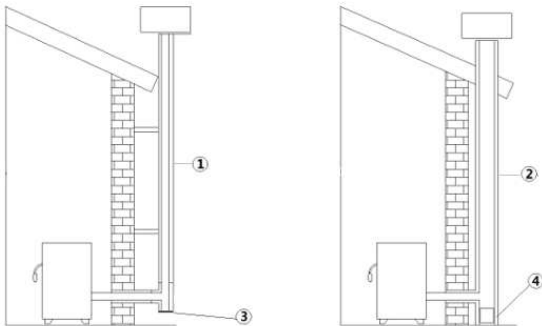
Fig. 3 - Rauchabzüge
