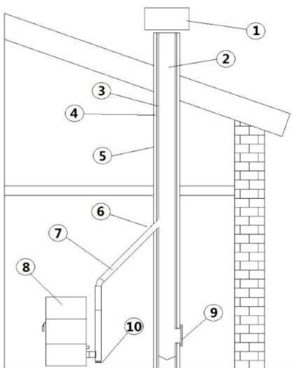
Fig. 2 - Bauteile Kamin
