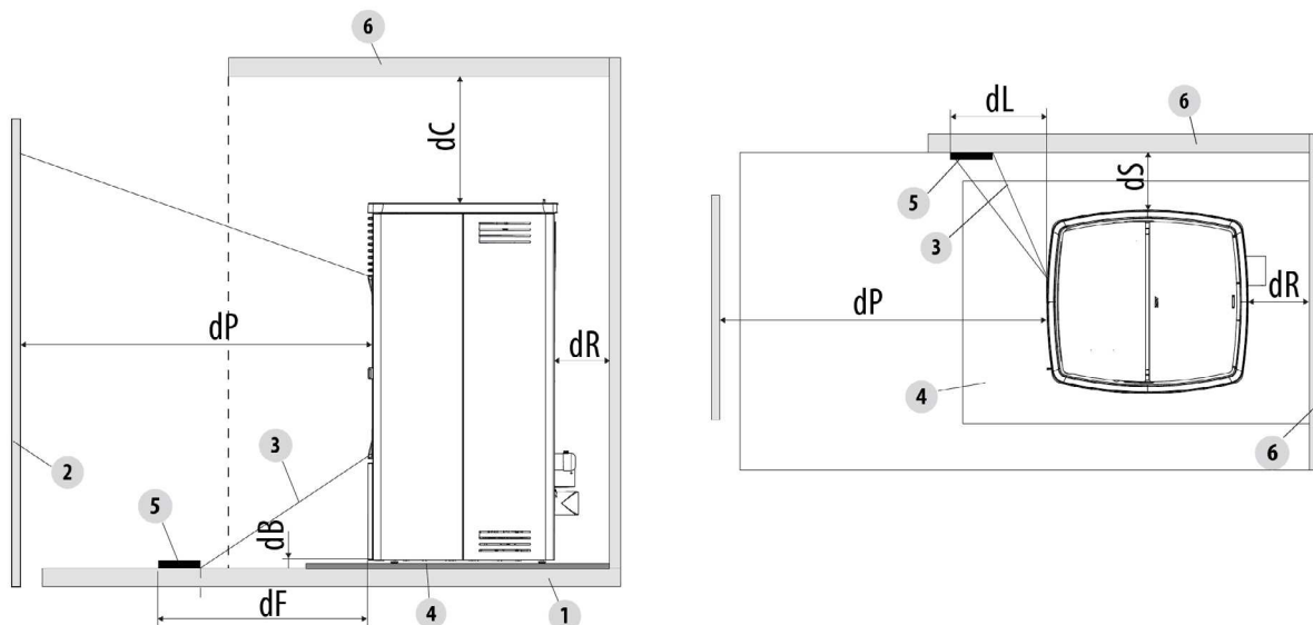
Fig. 11 - Sicherheitsabstand vom Brennstoff
