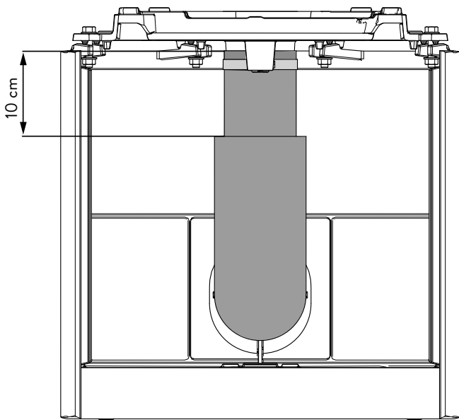
Abb. 12 - Sockel
