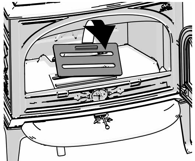
Afb. 24 Vervangen van asrooster
