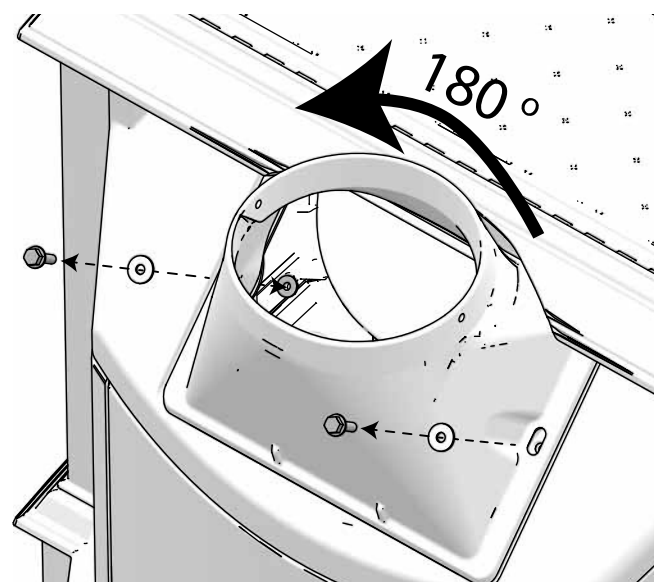
Afb. 5a Wisselen van boventuitlaat naar achteruitlaat
