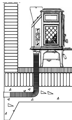
Rys. 7c Podłączenie wykonane przez podłogę i piwnicę
