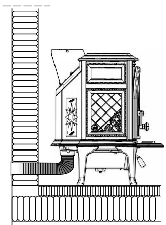
Abb.7a Durch eine Außenwand
